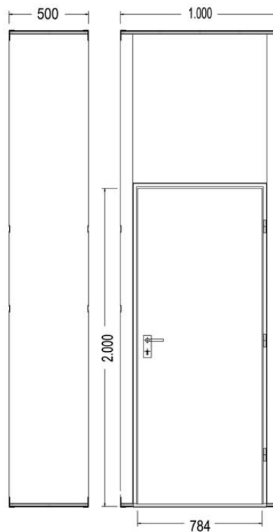
Türelement Ident-Nr.: 1504
